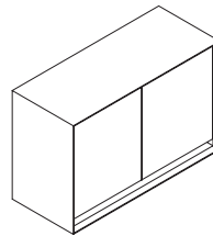
K1201DT77 Kommode mit 2 Türen, 1 Fachboden K601ET77 Chest with 2 doors, 1 shelve B 120, T 50, H 77 cm K1201DT100 Kommode mit 2 Türen, 2 Fachböden K1201DT100 Chest with 2 doors, 2 shelves B 120, T 50, H 100cm
